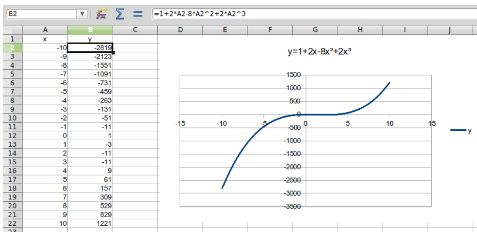
Figura 8.1: Ricerca delle radici di un'equazione per via grafica
