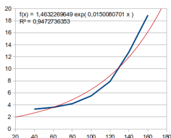
Figura 6.7: Grafici che illustrano il consumo di carburante in funzione della velocità
