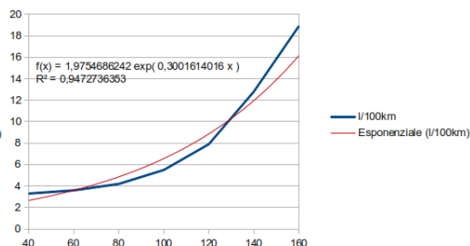
Figura 6.7: Grafici che illustrano il consumo di carburante in funzione della velocità
