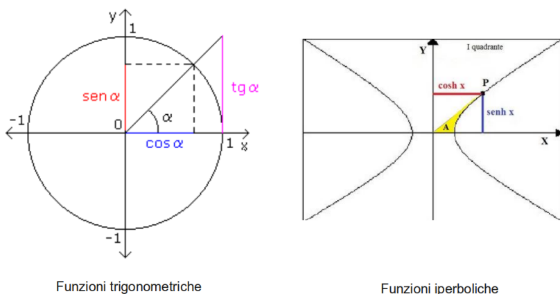
Figura 3.1: Differenza tra funzioni trigonometriche e funzioni iperboliche
