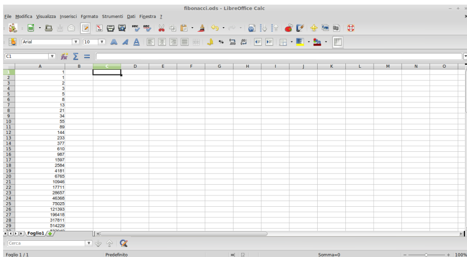
Figura 2.1: La successione di Fibonacci
